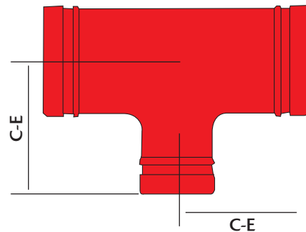
Trójnik redukcyjny - odejscie rowkowe, typ 7121
